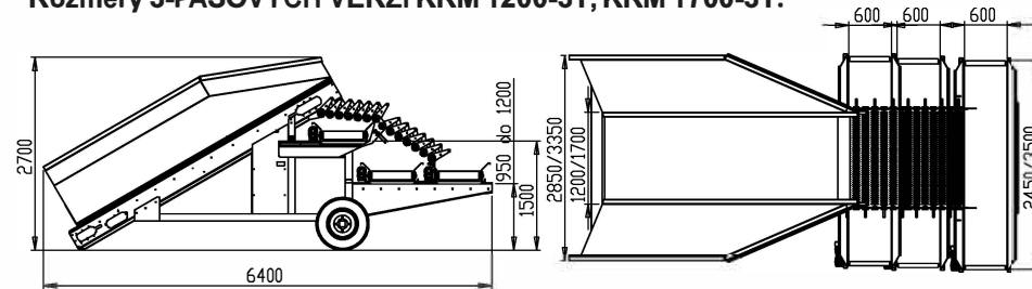
Rozměry 3-PÁSOVÝCH VERZÍ KRM 1200-3T, KRM 1700-3T:
