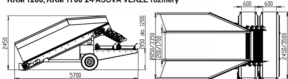
KRM 1200, KRM 1700 2-PÁSOVÁ VERZE rozměry
